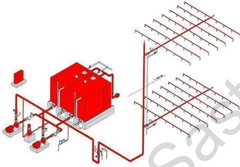
Şekil 4.8. Sprinkler sistemi.
